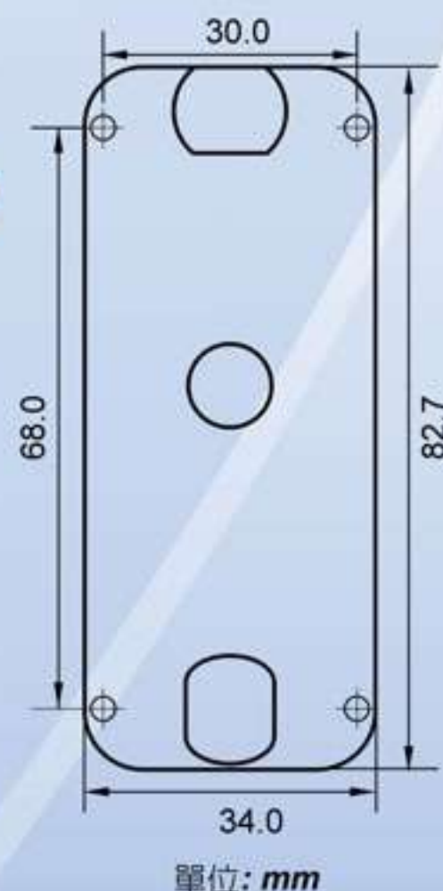
Mifare門禁控制器模組板 PIMF-C07
